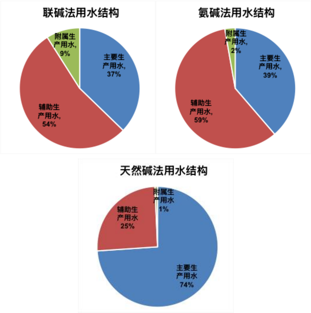
图 1 纯碱生产企业用水结构和主要用水环节示意图
