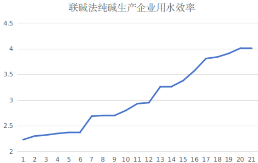
图 2 联碱法纯碱生产企业有效样本用水效率分布
