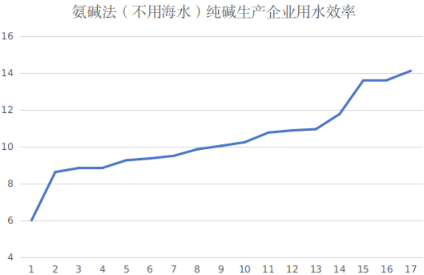
图 3 氨碱法（不用海水）纯碱生产企业有效样本用水效率分布
