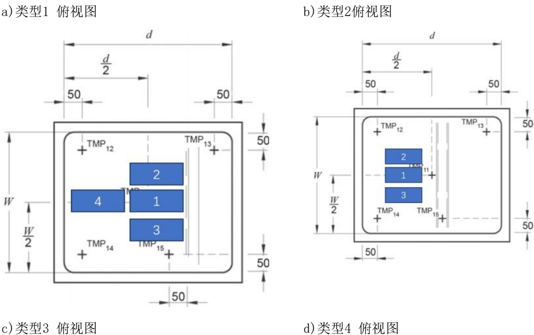
图1 卧式冷冻箱装载位置示意图
