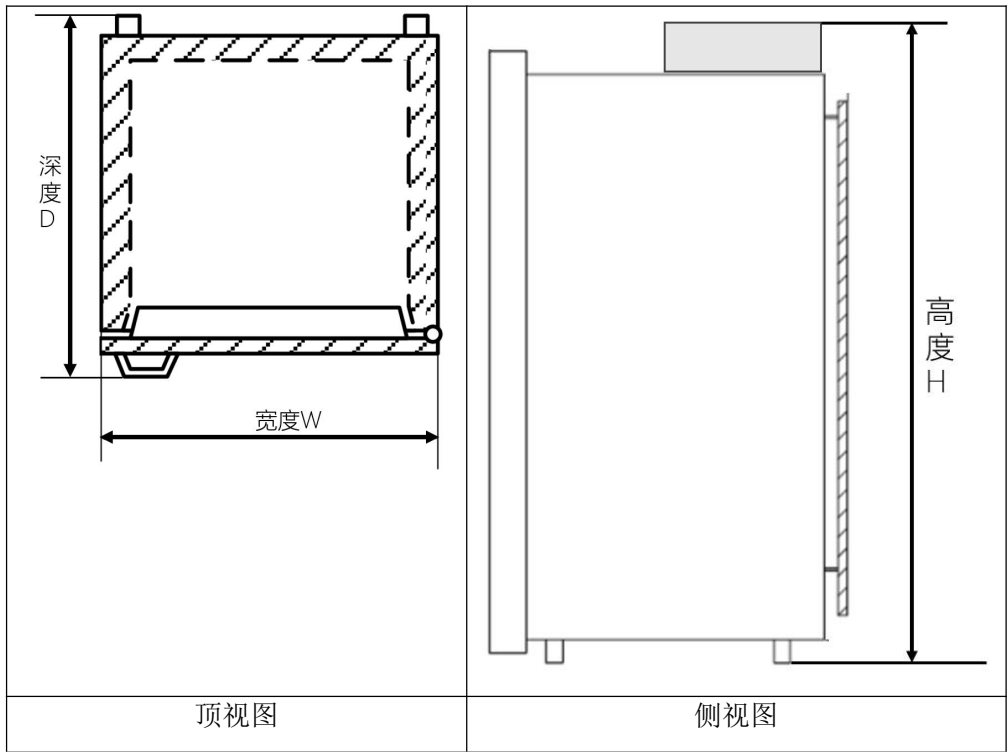
图2 外形体积测算时宽、高、深示意图
