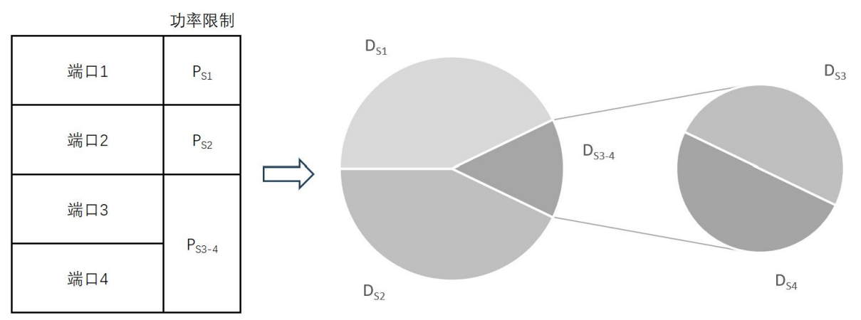
图 C.2 各端口功率限制比例示意图
