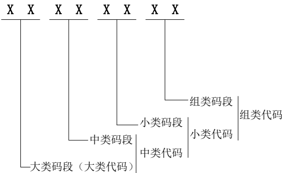
图1 代码结构
