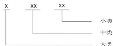
图1 代码结构图
